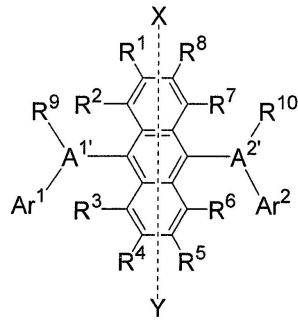
화학식 1'
