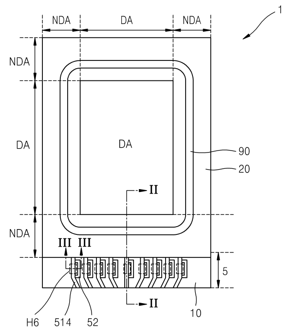
도면1
