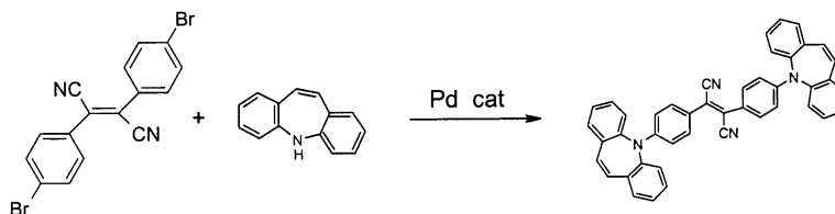
반응식 3
