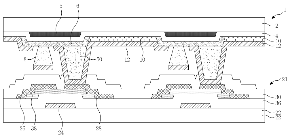
도면3
