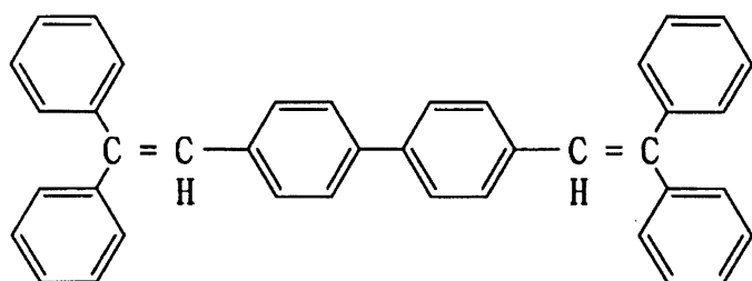
[화학식 5]
