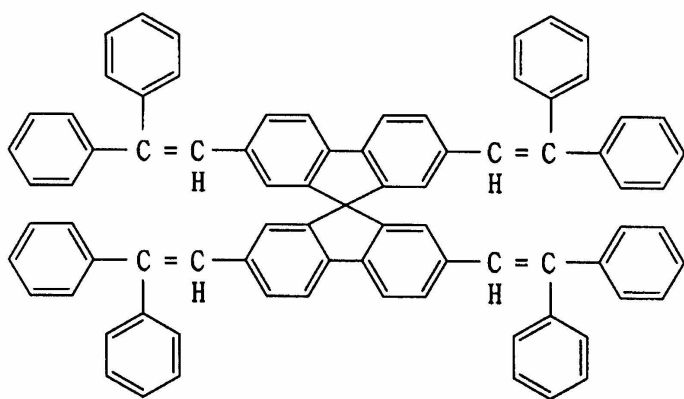
[화학식 8]
