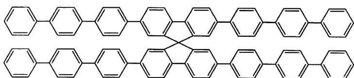
[화학식 9]
