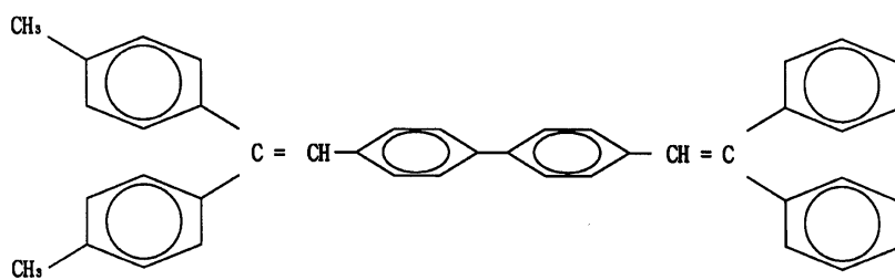
[화학식 4]
