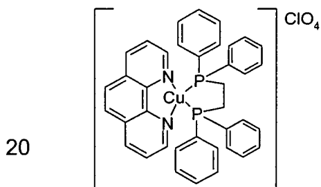
Emitter E1 (US 2005/0221115)
