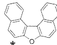
(IIe)
