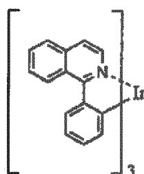
Ir(ppy) 3
