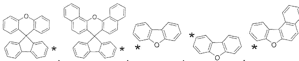
(IIa)
