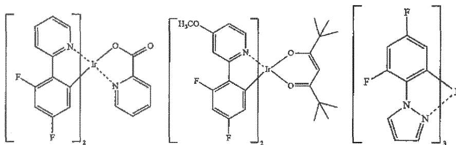
F_2Irpic
