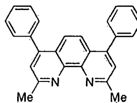
BCP
