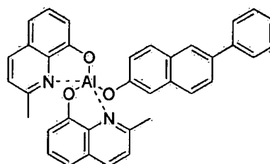
BAiq 유도체
