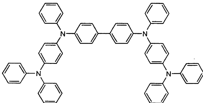
TPD232
