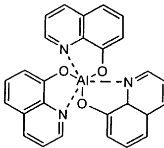
Alq
