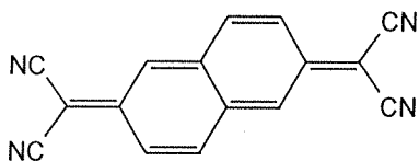
TNAP
