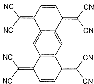
OCNAQ
