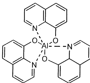
Alq
