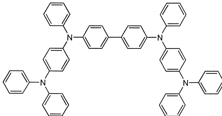
TPD232
