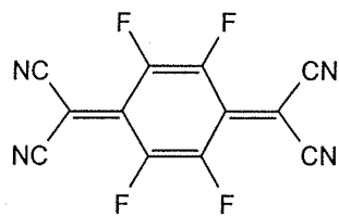
TCNQ-4F
