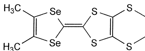
DMET
