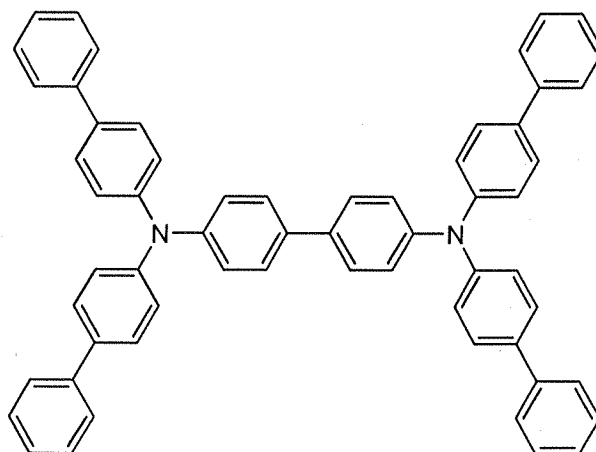
TBDB
