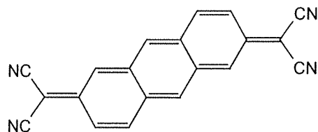
TNAT
