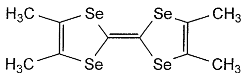
TMTSF
