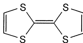
TTF
