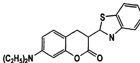
coumarin 6
