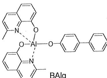
BAlq
