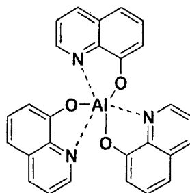
Alq
