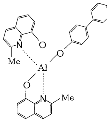
BAlq
