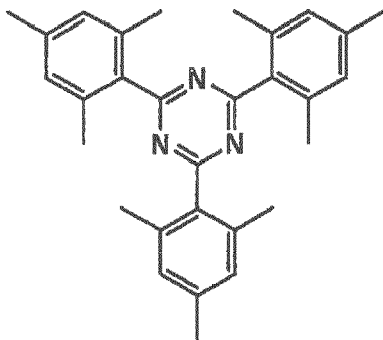
D1-3
