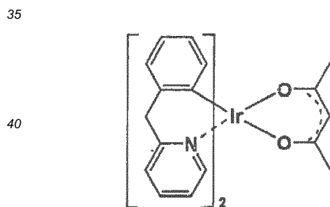
D-3
