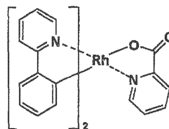
D-6
