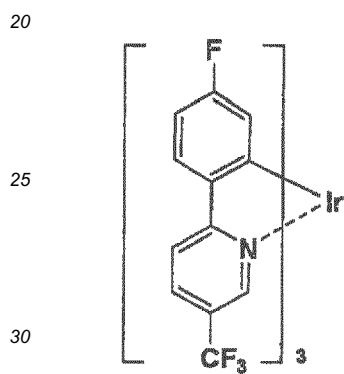
D-1
