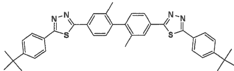
A1-7
