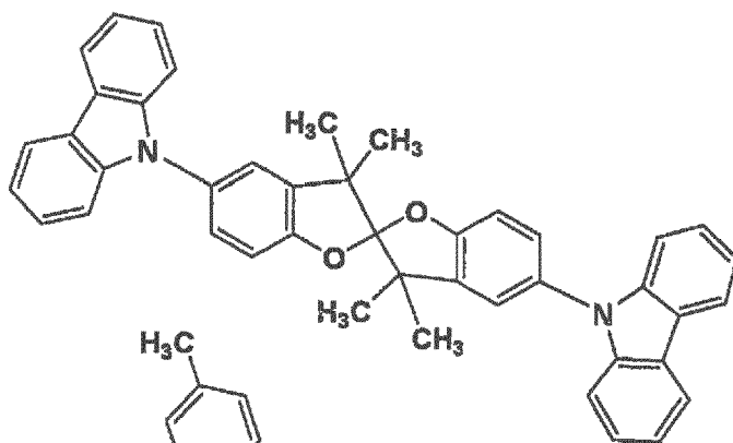
JA-7
