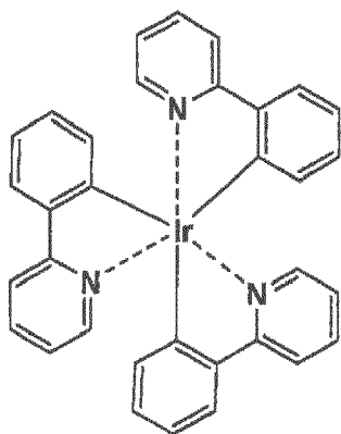
Ir-3
