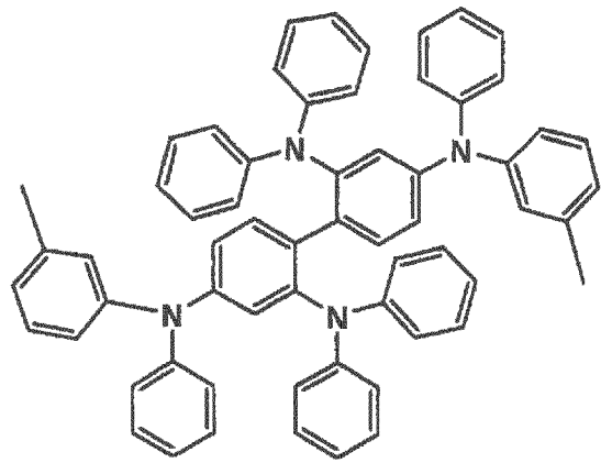
C-20
