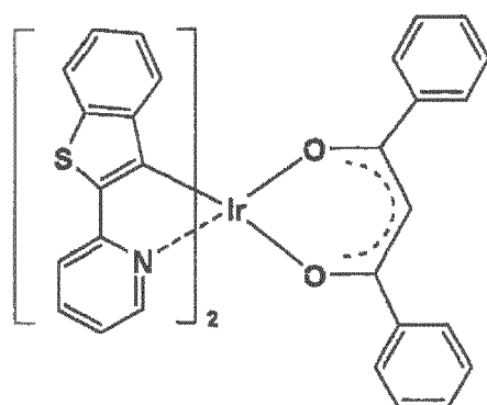
Ir-9
