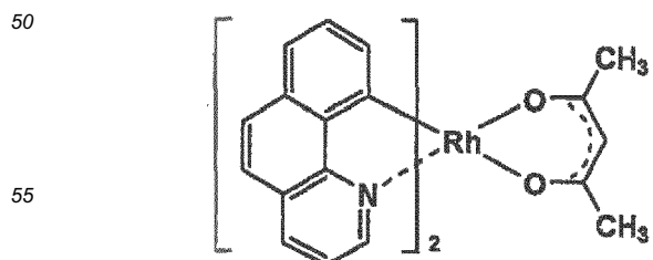
D-5
