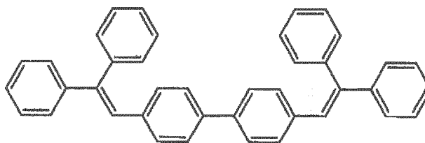
(DPVBi)
