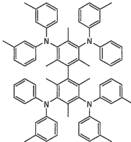
C-22
