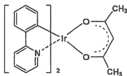
Ir-10
