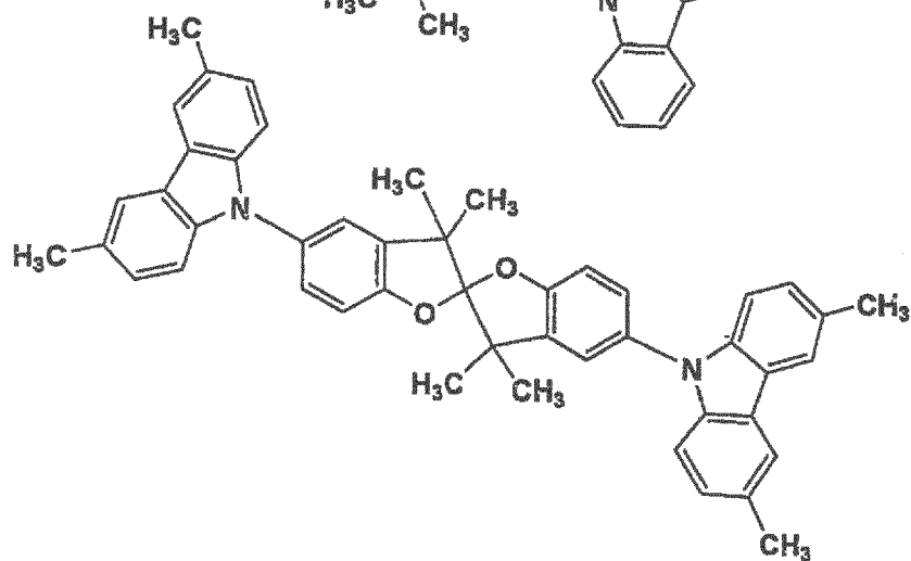
HC1
