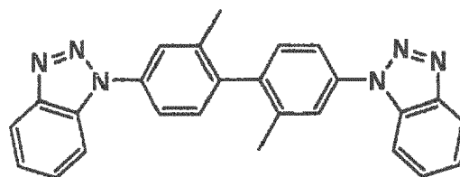
A2-1
