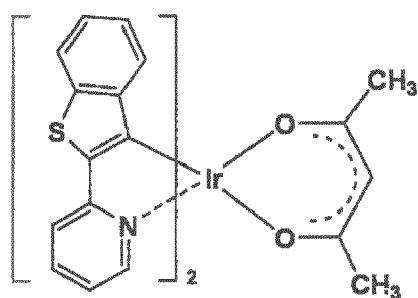
Ir-11
