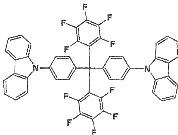
HC7
