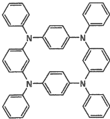
C-21
