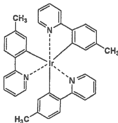
Ir-4
