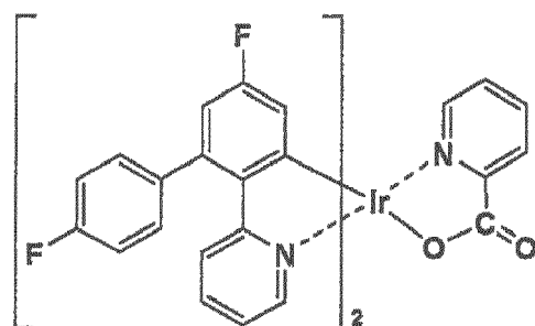
Pt-2
