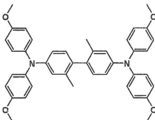
C-23
