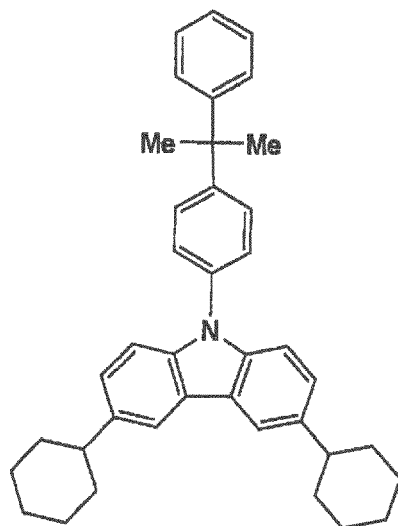
11-18
