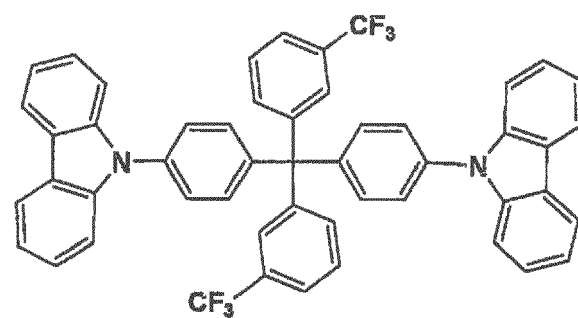
HC9
