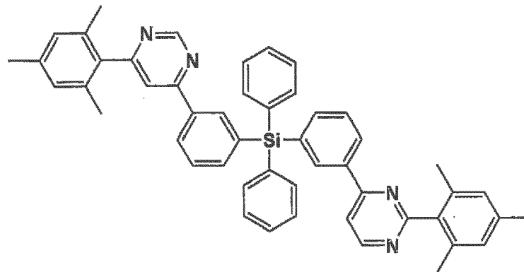
A1-6
