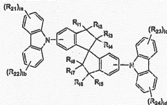
Formula I1
