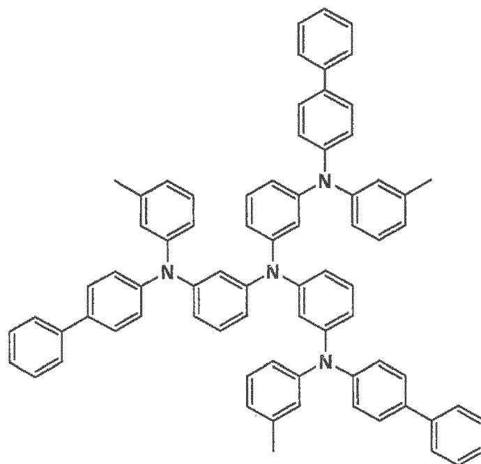
C-18
