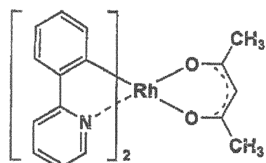
D-6
