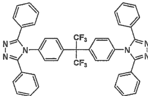
A3-1
