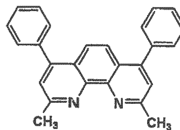
BCP
