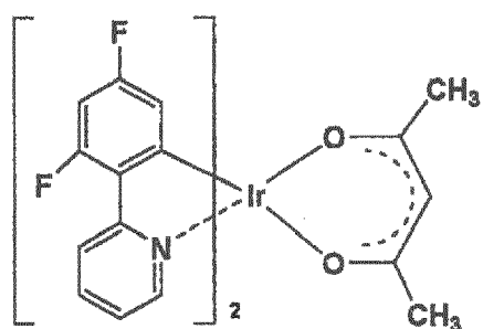
Ir-12
