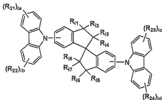
Formula I1
