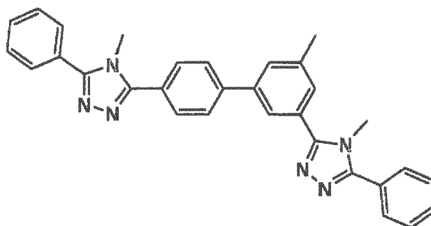
A1-4
