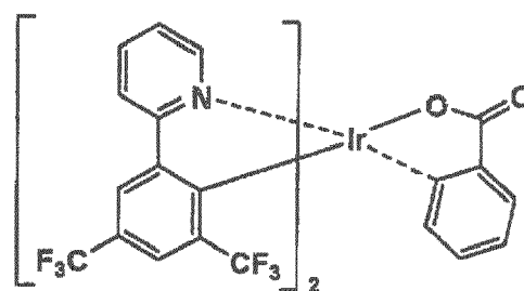
D-4
