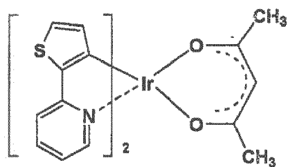
Ir-7
