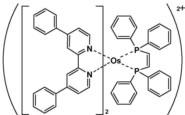
A-1
