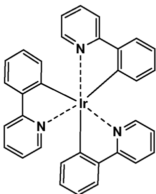
Ir-3
