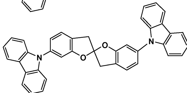
JA-6
