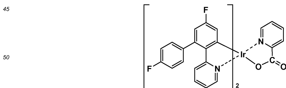
Ir-13
