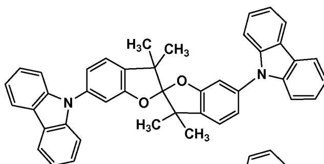
JA-5
