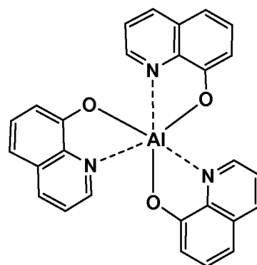
Alq 3
