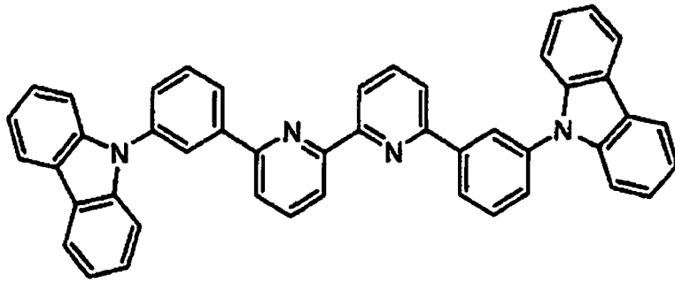
[Chemische Formel 95]
