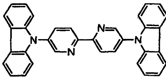
[Chemische Formel 97]
