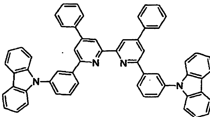
[Formule chimique 101]
