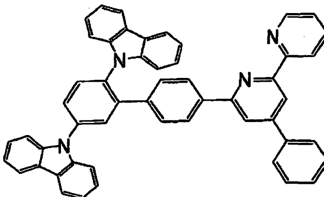
[Chemische Formel 103]
