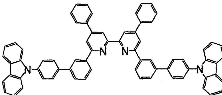
[Chemische Formel 102]
