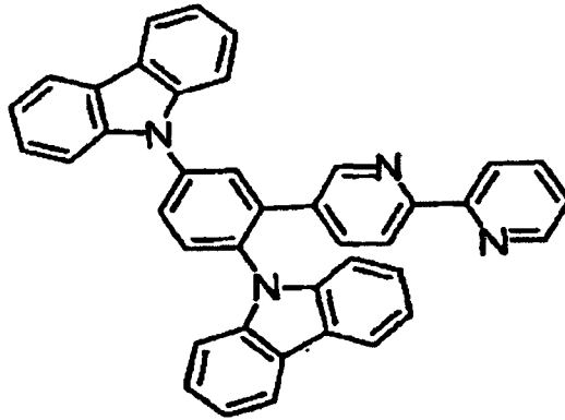
[Chemische Formel 98]
