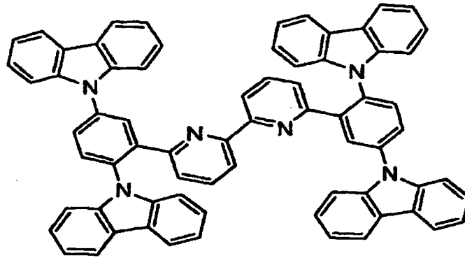
[Formule chimique 96]
