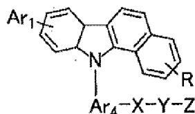
Chemische Struktur 5
