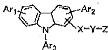
Chemische Struktur 6
