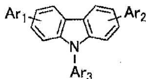
Chemische Struktur 1
