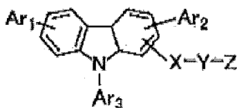
Structure chimique 6
