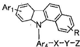
Structure chimique 5
