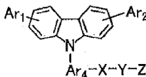
Chemische Struktur 3
