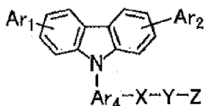
Structure chimique 3
