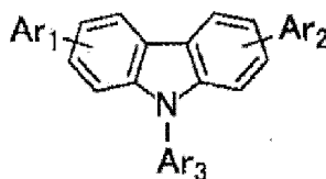
Structure chimique 1
