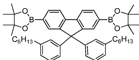
Monomer G
