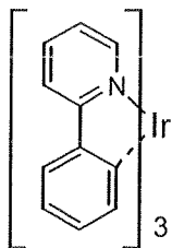
Ir(ppy) 3
