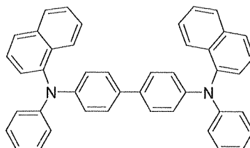
\alpha -NPD
