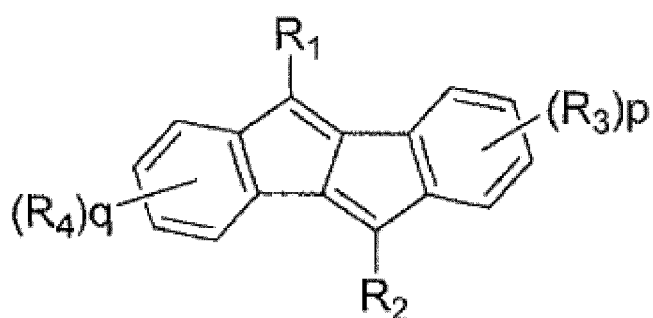
[Formule chimique 9]
