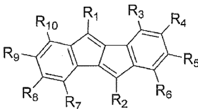
[Formule chimique 1]
