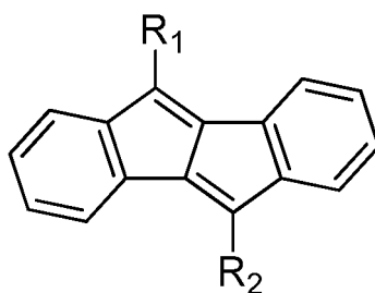
[Chemische Formel 3]
