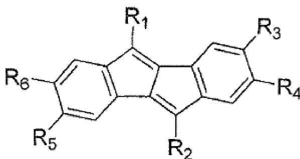
[Formule chimique 3]
