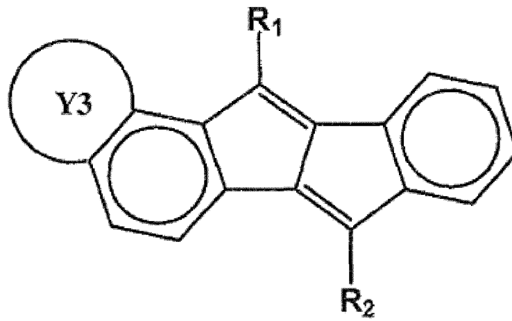
[Formule chimique 6]
