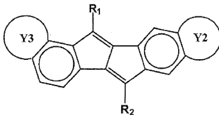
[Formule chimique 8]
