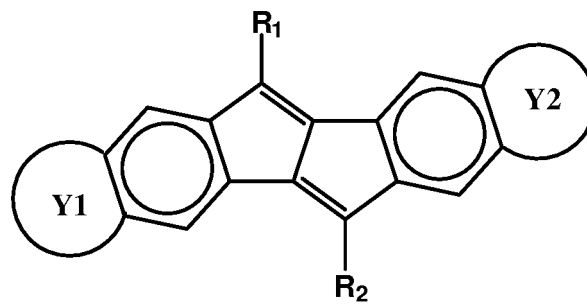
[Chemische Formel 6]
