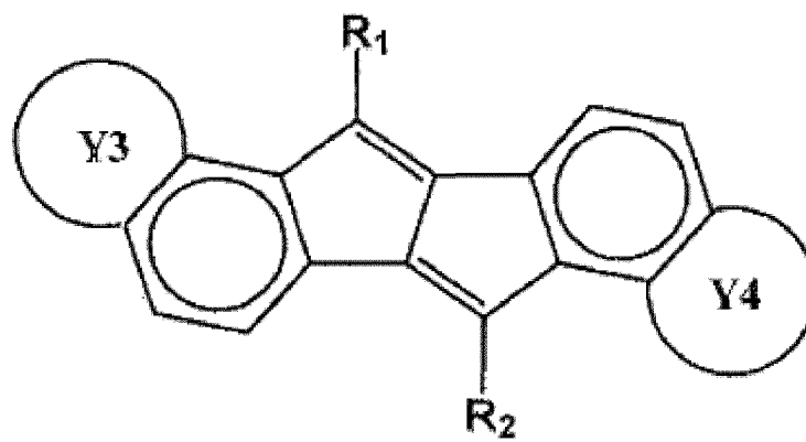
[Formule chimique 7]
