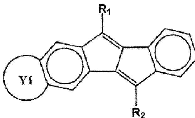
[Formule chimique 4]
