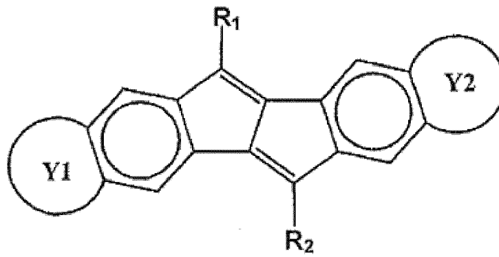
[Formule chimique 6]
