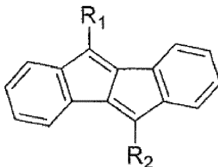
[Formule chimique 2]
