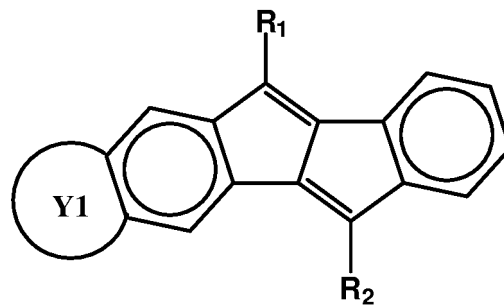
[Chemische Formel 5]
