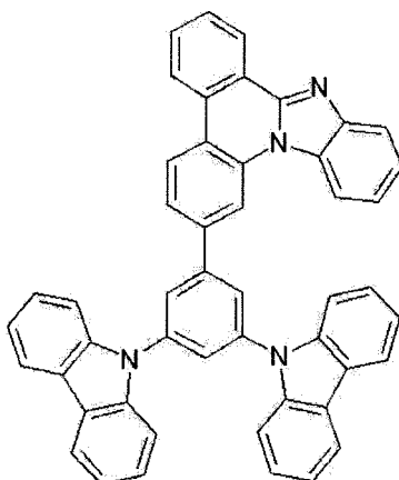
[GH]
