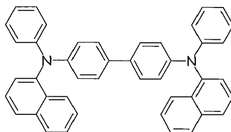
\alpha -NPD
