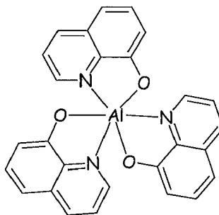
Alq 3
