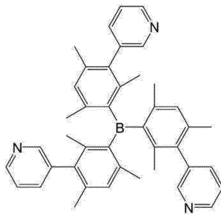
3TPYMB
