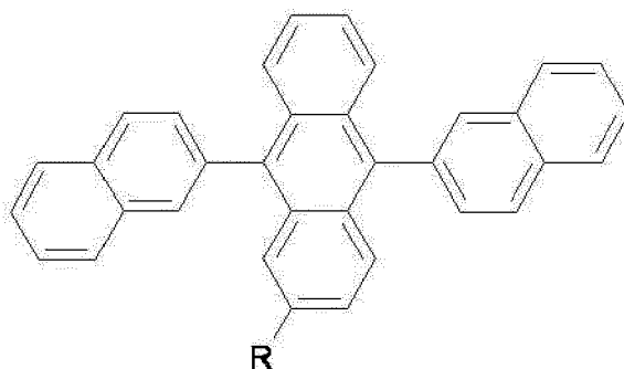
DNA/MADN/TBADN
