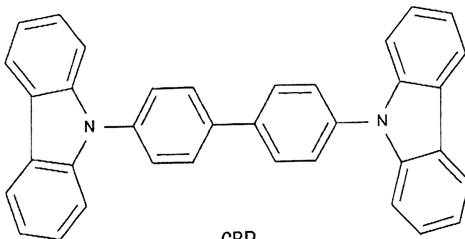
CBP
