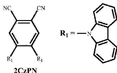
3-CzTRZ: (3'-(4,6-diphenyl-1,3,5-triazin-2-yl)-(1,1'-biphenyl)-3-yl)-9-carbazole
