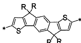
(V-14)
