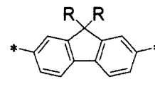
(V-9)
