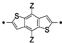
(V-7)
