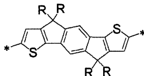
(V-14)
