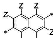
(V-8)
