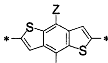
(V-7)
