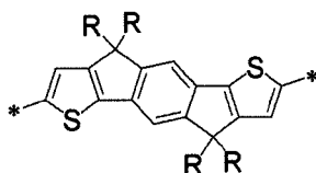
(V-14)
