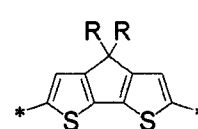
(V-5)
