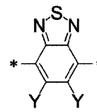
(V-16)
