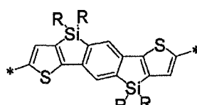
(V-15)
