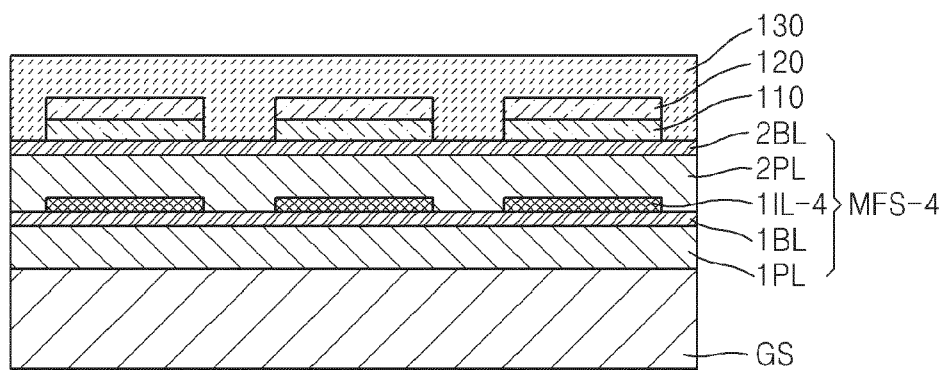
FIG. 15B
