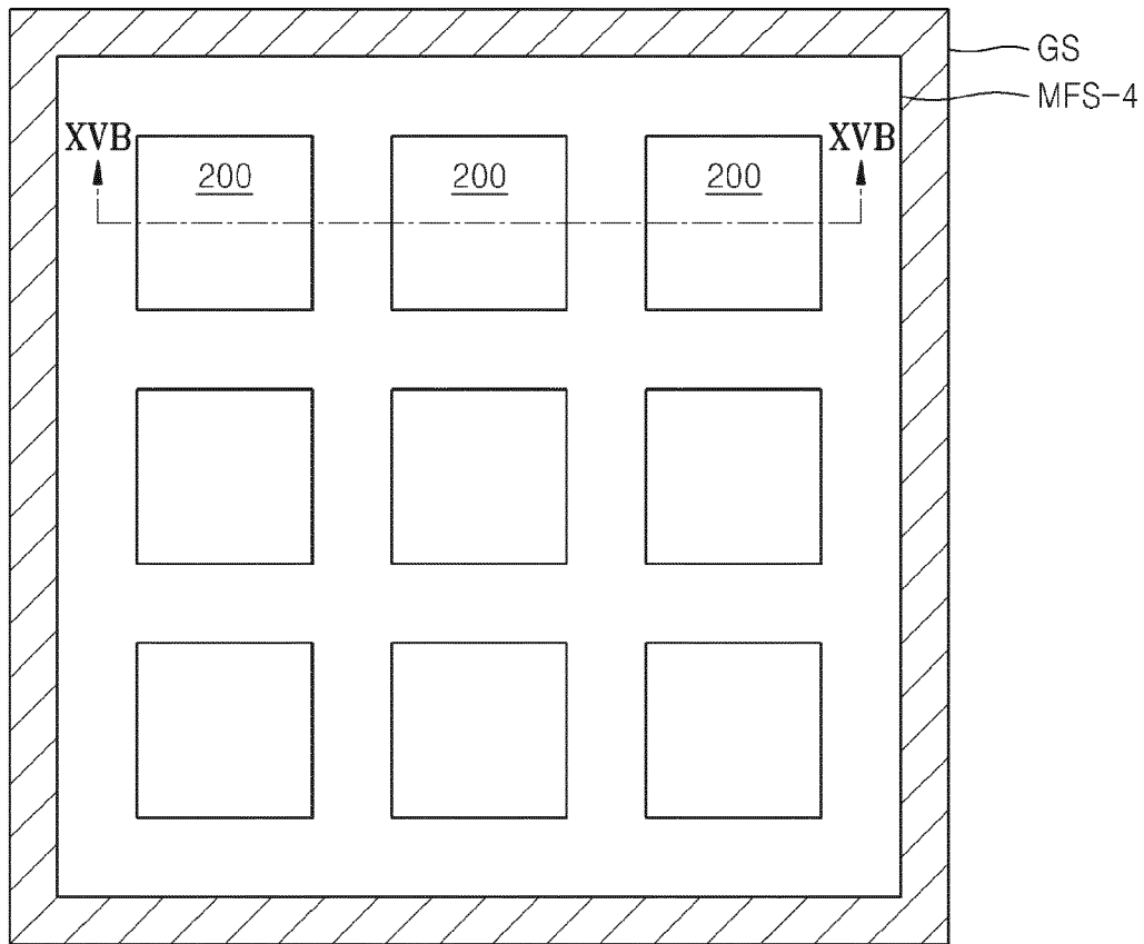
FIG. 15A
