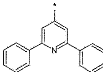
[Formule chimique 9]
