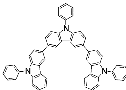
Tris-PCz
