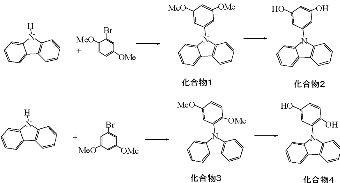
スキーム 1
