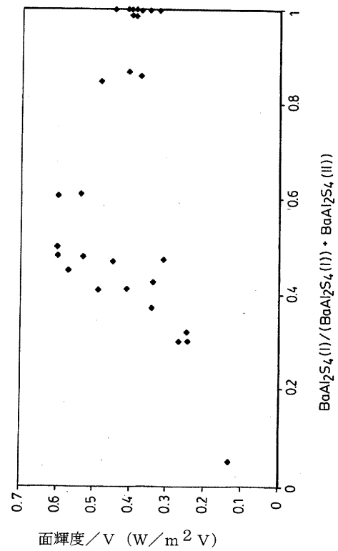
FIG. 10. BaAl 2 S 4 の全体に対するBaAl 4 S 7 (I) の比を関数とする輝度傾斜
