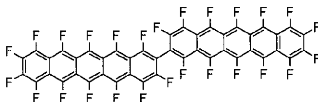
化合物 M ( C_{44}F_{26} )
