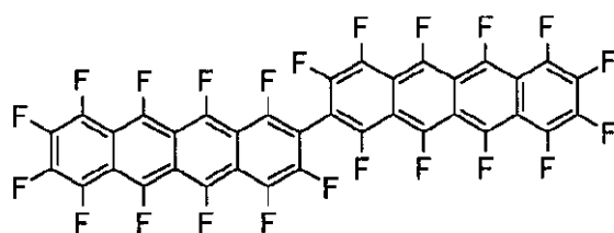
化合物 L ( C_{36}F_{22} )
