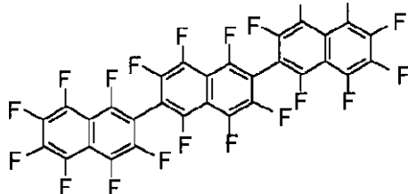
化合物 I ( C_{30}F_{20} )
