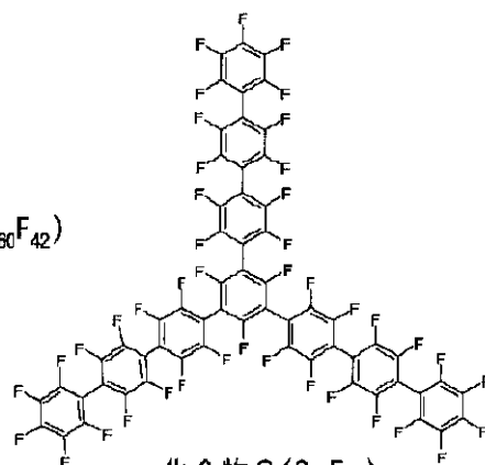
化合物C (C 60 F 42 )
