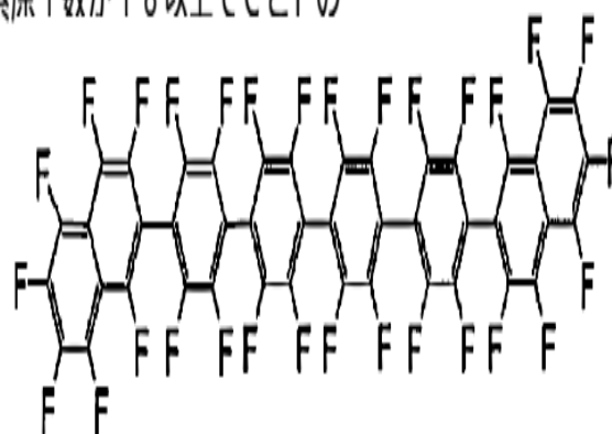
化合物G (C 44 F 30 )
