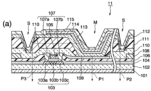
IV(a)-IV(a)断面図
