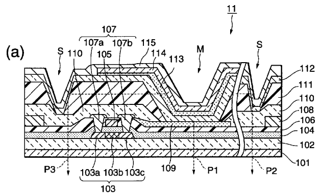
IV (a)-IV (a)断面図
