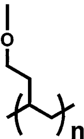
一般式(12)
