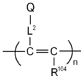
一般式(11)
