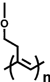
一般式(13)
