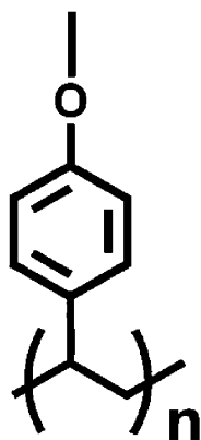
一般式(14)
