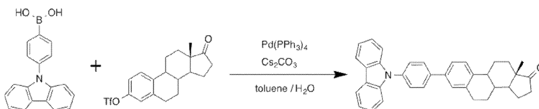
化合物 1
