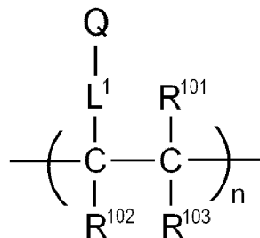
一般式(10)
