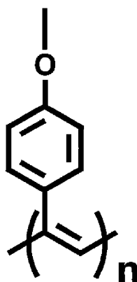
一般式(15)
