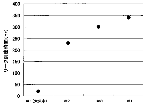
発光素子リーク破壊への到達時間
