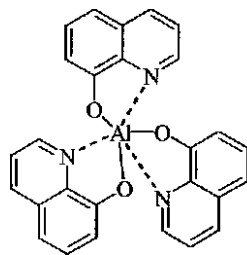
トリス(8-キノリノール)アルミニウム
