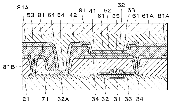
図17B [工程 - 330](続き)
