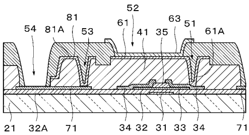
図13B [工程 - 220](続き)
