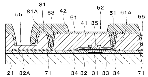
図18B [工程 - 400]つづき
