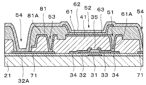
図14B [工程 - 220](続き)
