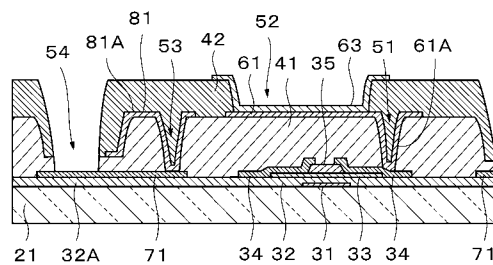
図19B [工程 - 410](続き)
