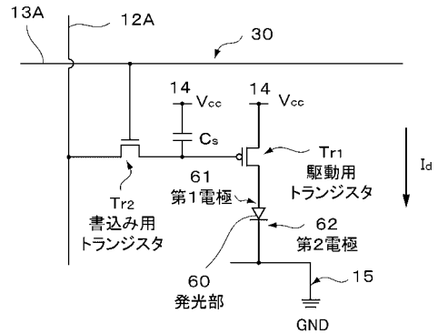
図2B Tri:n-チャンネル型
