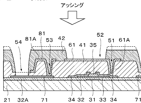
図19A [工程 - 410](続き)
