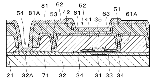
図20B [工程 - 410](続き)
