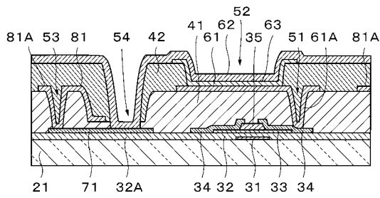
図17A [工程 - 330](続き)
