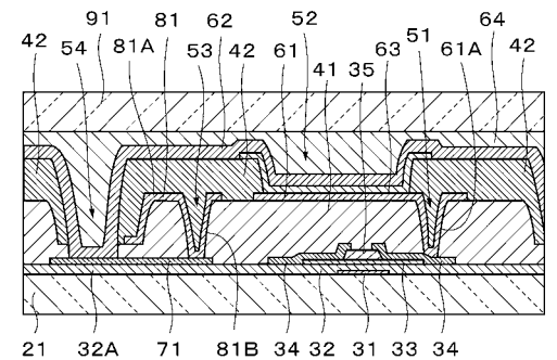
図20B [工程 - 410](続き)
