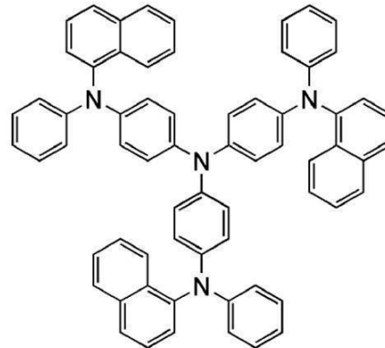
1'-TNATA
