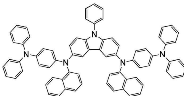
PCzTPN2
