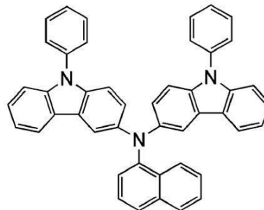
PCzPCN1
