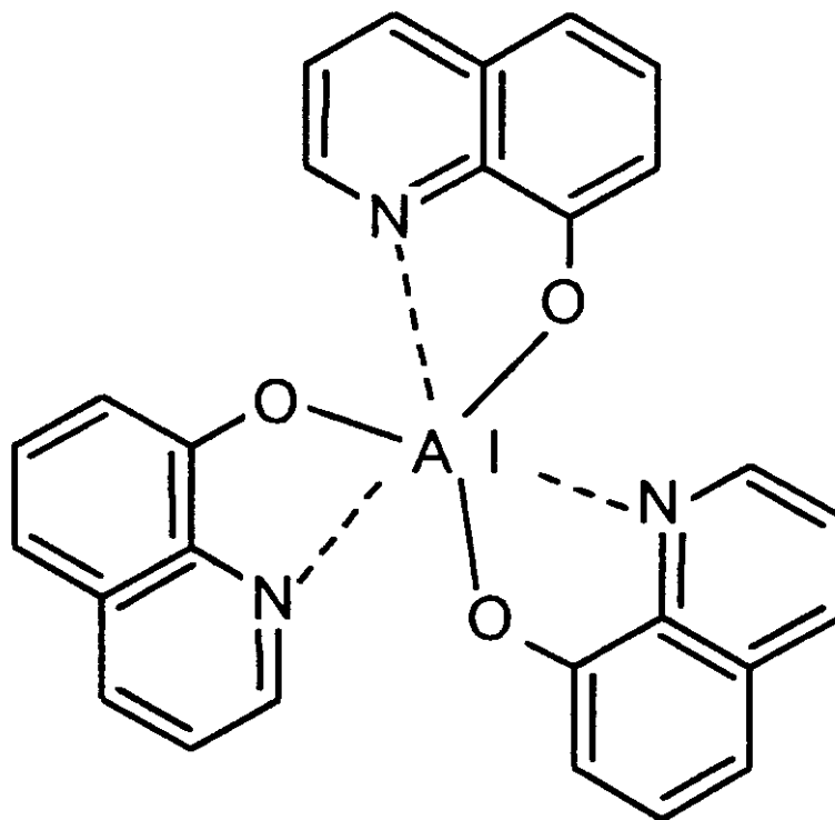
Alq 3
