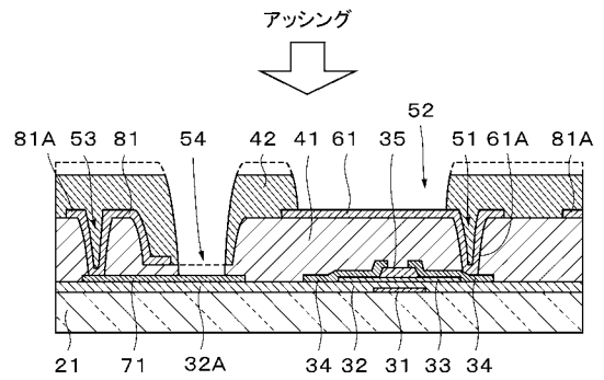
図16A [工程 - 320]
