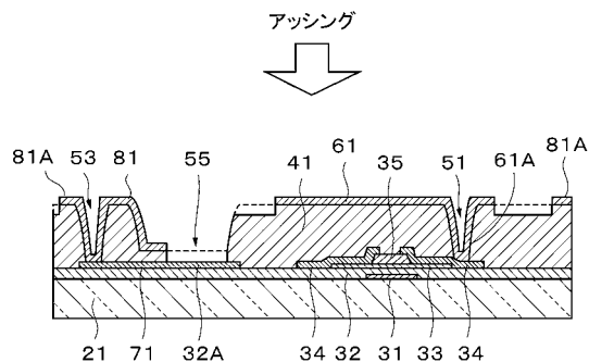
図8B [工程 - 140]
