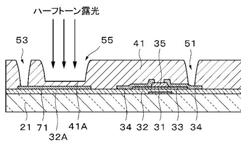
图7A [工程-120]
