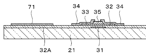
図6C [工程 - 100](続き)
