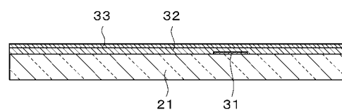
図6A [工程 - 100]
