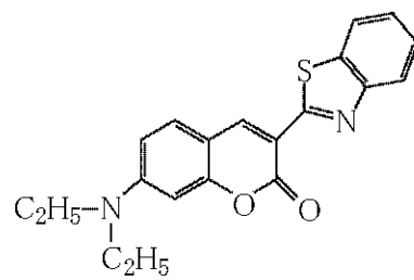
comarin6
