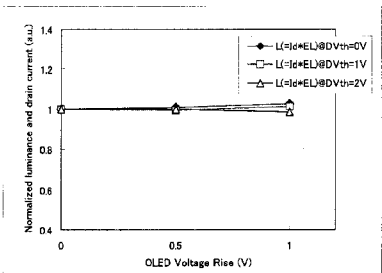
実施例2の画素回路の画素輝度計算例 (EL vs ΔV: DCJTb @65C [Ref.3])
