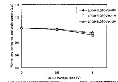
実施例2の画素回路の画素輝度計算例 (EL vs ΔV: C545T @22C [Ref.3])
