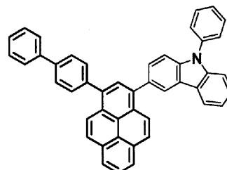
化合物[15]
