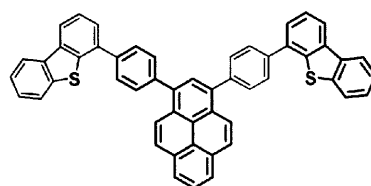
化合物[24]
