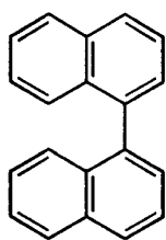
1,1'-ビナフチル
