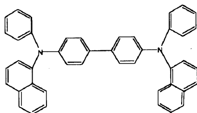
\alpha -NPD
