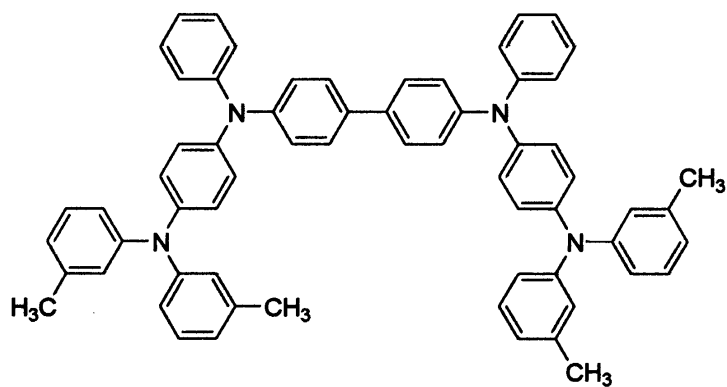
DNTPD
