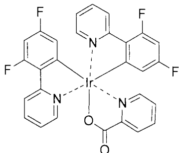
化合物 ( E )
