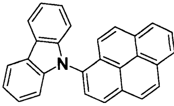
化合物 (A)
