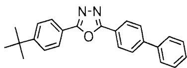
化合物（G）
