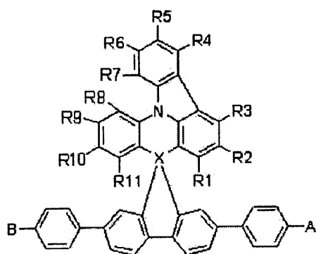
〔化学式3〕
