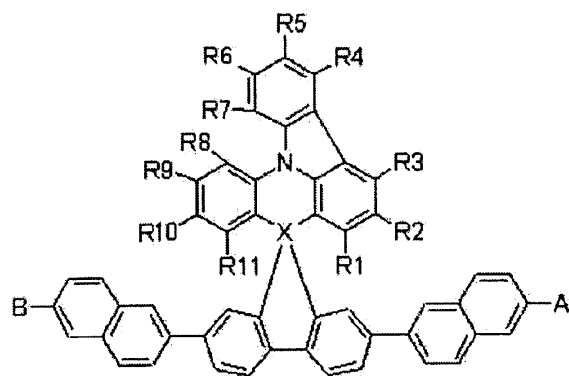
〔化学式4〕
