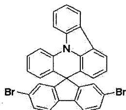
[化学式 b]
