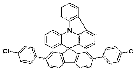
[化学式 c]
