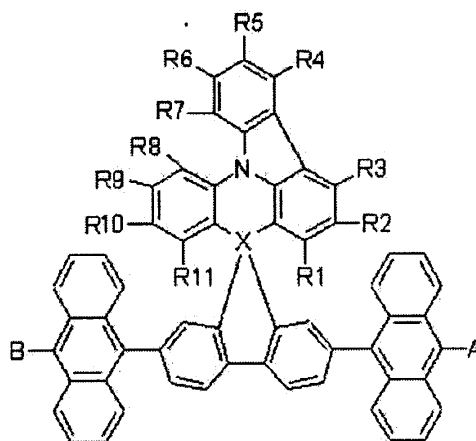
〔化学式5〕
