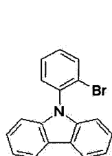
[化学式 a]
