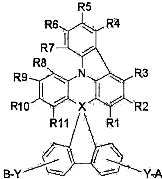
〔化学式 1〕
