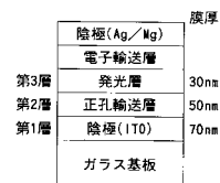
図101 有機EL素子の構成断面図
