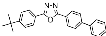
化合物 (G)
