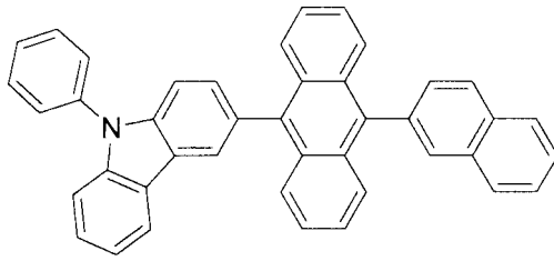
化合物 (C)
